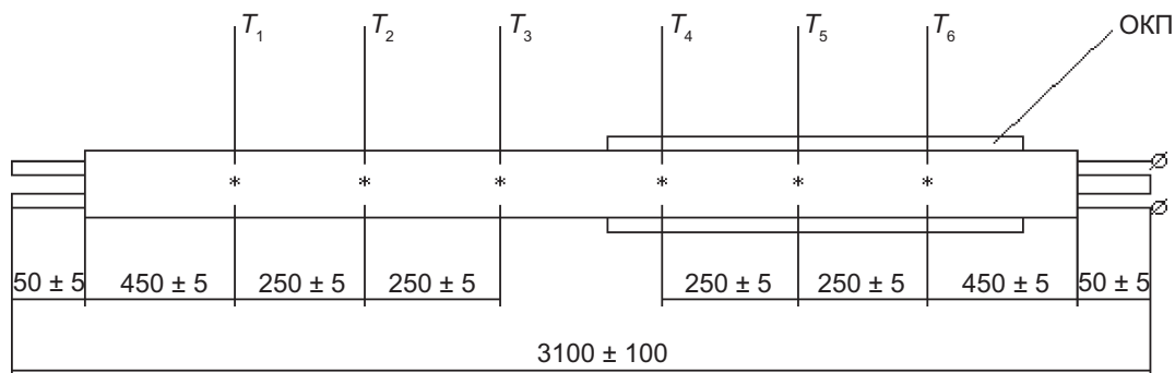
Рис. 1 — Размещение термоэлектрических преобразователей
